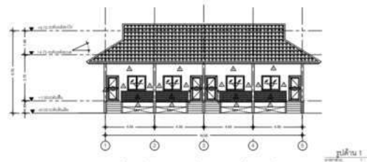
รูปด้าน 1
