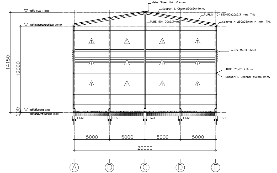
รูปตัด B-B 2/002 SCALE 1:300
