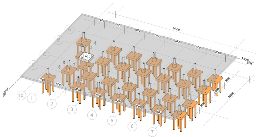
1 ฝั่งฐานรากจากเสาเข็มแบบ 3 ฝิต
