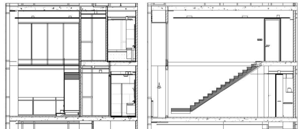
ความคืบหน้าแบบจำลองข้อมูลอาคารงานสถาปัตย์ภายใน : ห้อง Duplex
