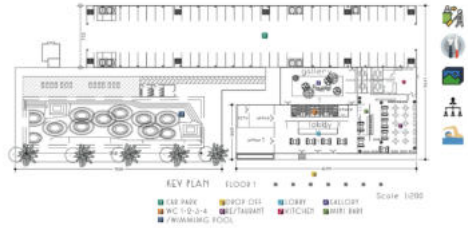
ภาพที่ 4 : ผังบริเวณชั้นที่ 1
