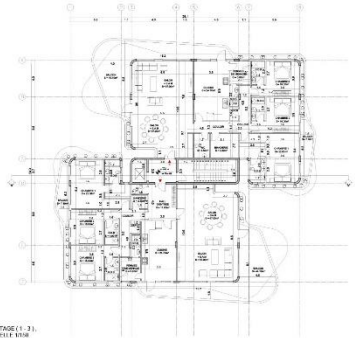
PLAN ETAGE (1-2) Echelle: 1/500
