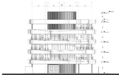
FACADE BLD Echelle: 1/100
