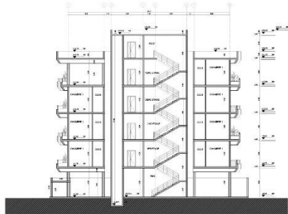
Coupe AA Echelle: 1/100
