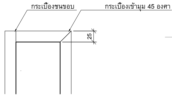
E1 A5-01 SCALE 1:10 แบบขยาย E1
