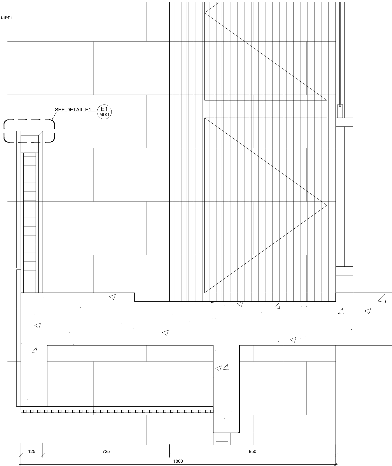
F A5-01 SCALE 1:10 แบบขยายที่ผนังระเบียง
