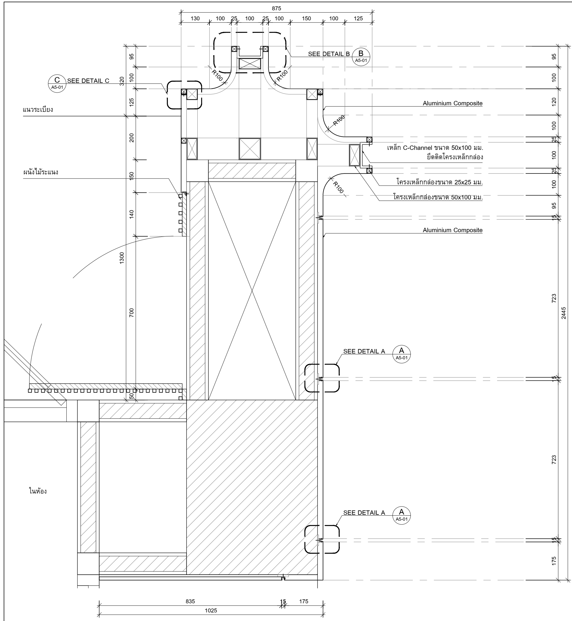
3 A5-01 แบบขยาย FACADE 3 SCALE 1:10
