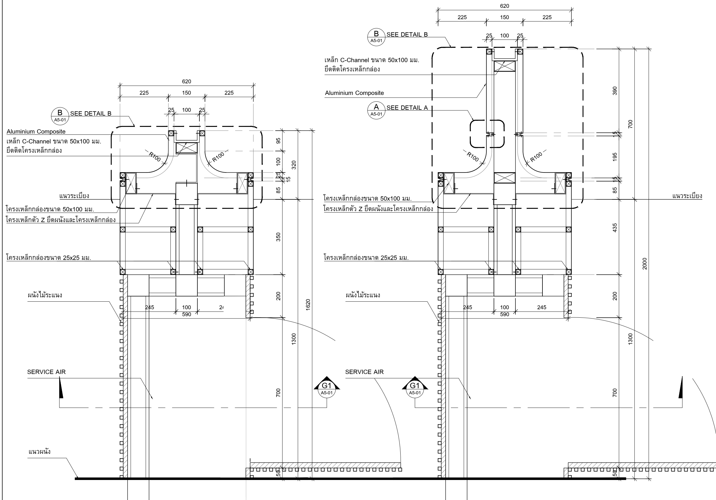
1 แบบขยาย FACADE 1 A5-01 SCALE 1:10
