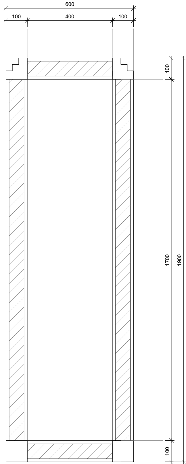
X A5-01 SCALE 1:10 แบบขยาย X
