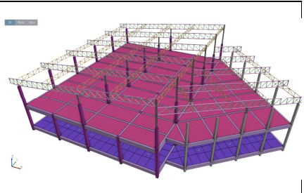
อาคารโรงงานเบเกอร์รี่ 2 ชั้น
