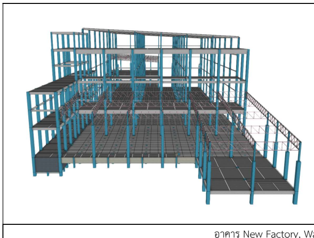
อาคาร New Factory, Warehouse (ASRS) และ Office
