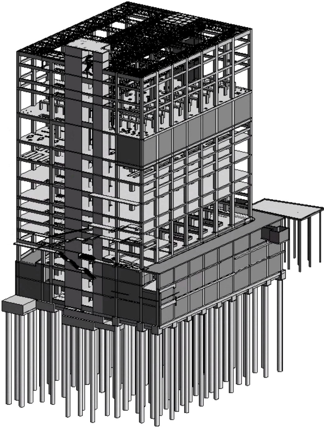
รูปที่ 14 แบบจำลอง REVIT 3D
