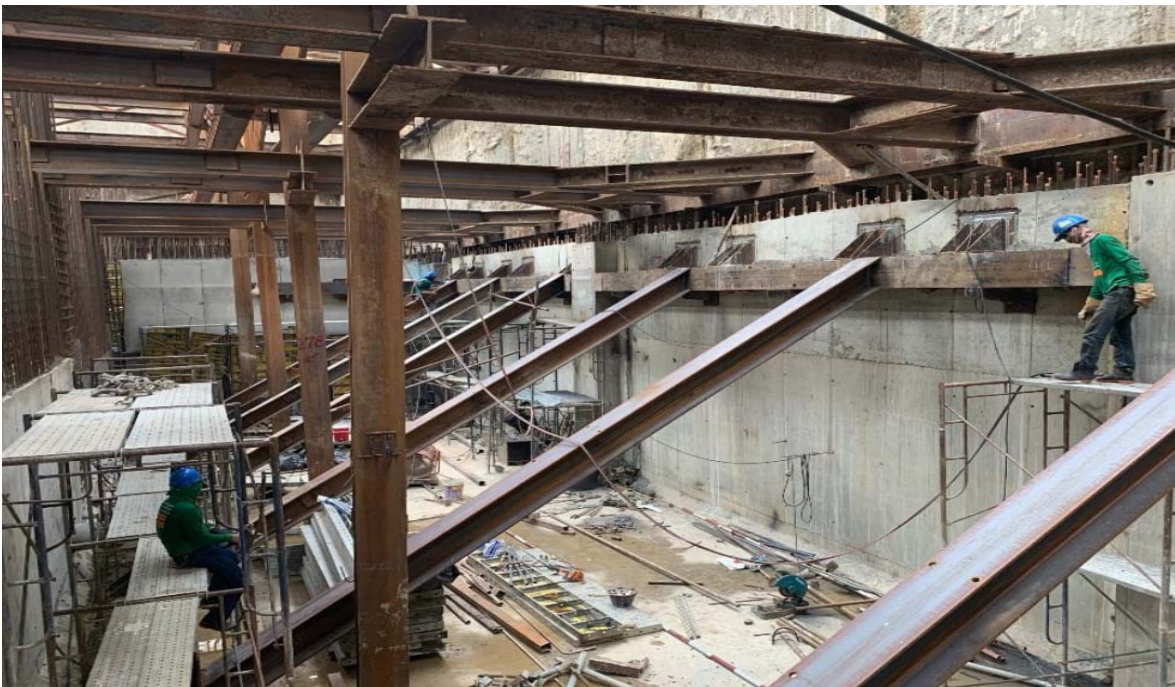
รูปที่ 11 งาน โครงสร้างค้ำยัน
