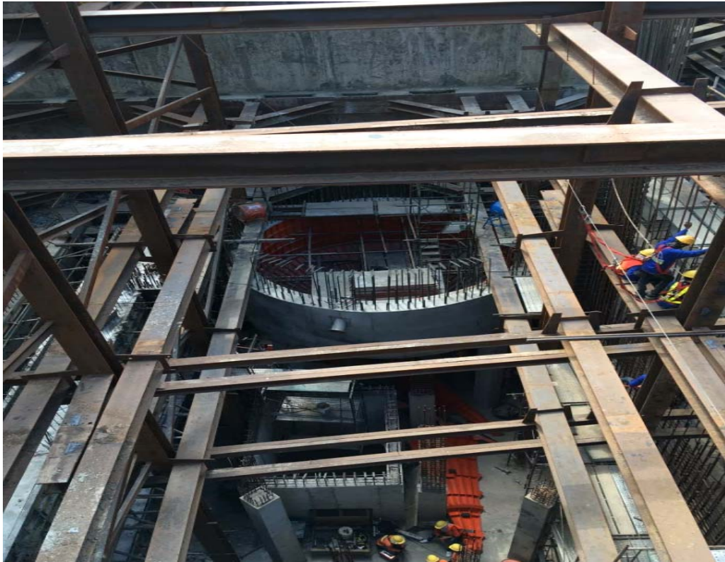
รูปที่ 13 งาน โครงสร้างถังไซโต
